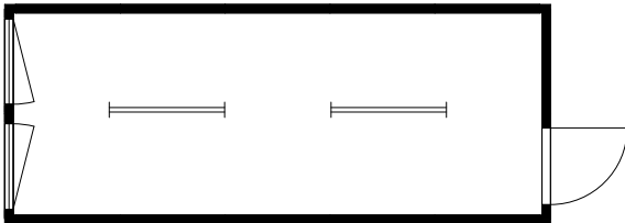
20f Aufenthaltscontainer 6.055 x 2.435 x 2.800mm
