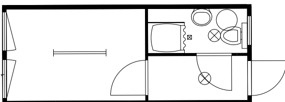
20f Aufenthaltscontainer inkl. Duschabteil 6.055 x 2.435 x 2.800mm
