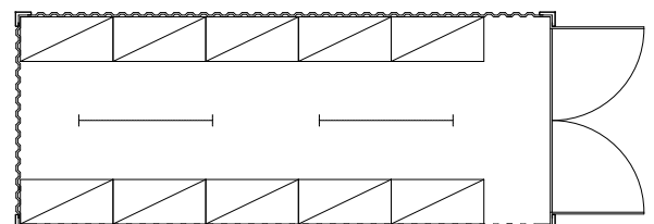
20f Lagercontainer inkl. beidseitigen Schwerlastregalen 6.058 x 2.438 x 2.591mm
