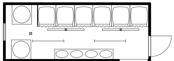
20f Duschcontainer inkl. Windfang 6.055 x 2.435 x 2.800mm
