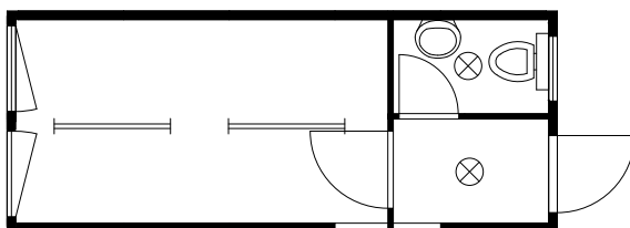
20f Aufenthaltscontainer inkl. WC-Abteil 6.055 x 2.435 x 2.800mm
