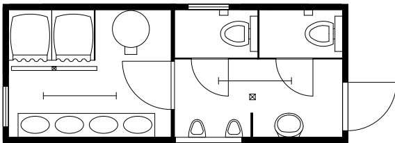
20f Toilett-/Waschcontainer Vorraum mit WC und abgetrenntem Waschbereich 6.055 x 2.435 x 2.800mm
